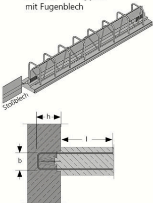
COMAX® WU Typ S1 mit Fugenblech
