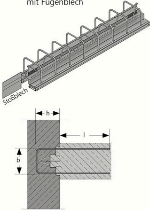
COMAX® WU Typ S1 mit Fugenblech
