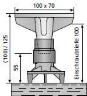
Kobold® B 15 (ohne) / mit Distanzhülse
