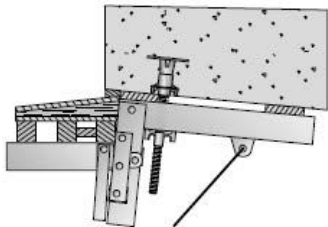
Kobold® B 15 (ohne) / mit Distanzhülse
